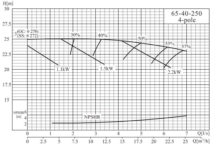
NISO, NIS, NISF 65-40-250/65-40-315
