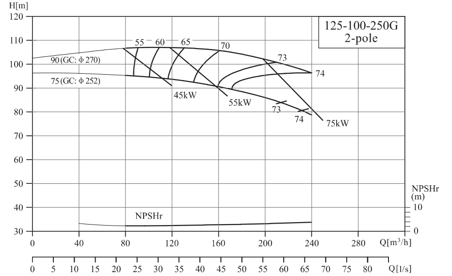
NIS125-100-250G/125-100-315G
