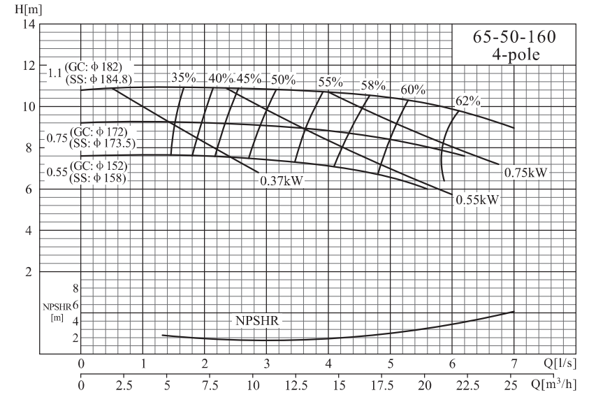
NISO, NIS, NISF 65-50-160/80-50-200
