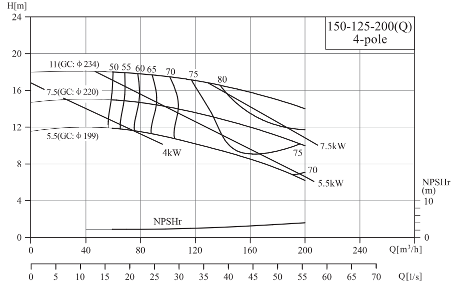
NIS150-125-200(Q)/150-125-200G
