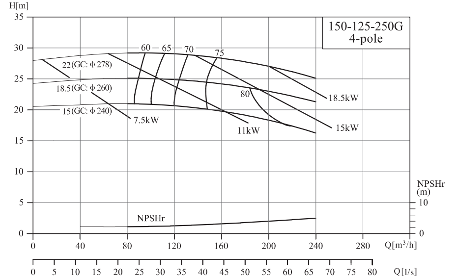
NIS150-125-250G/150-125-315(Q)
