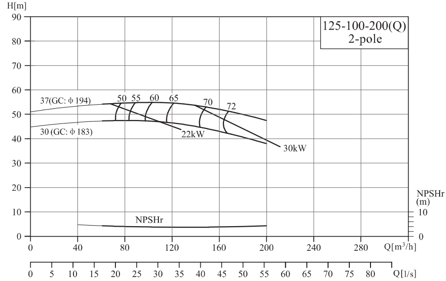
NIS125-100-200(Q)/125-100-200G
