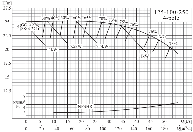
NISO, NIS, NISF 125-100-250/125-100-315
